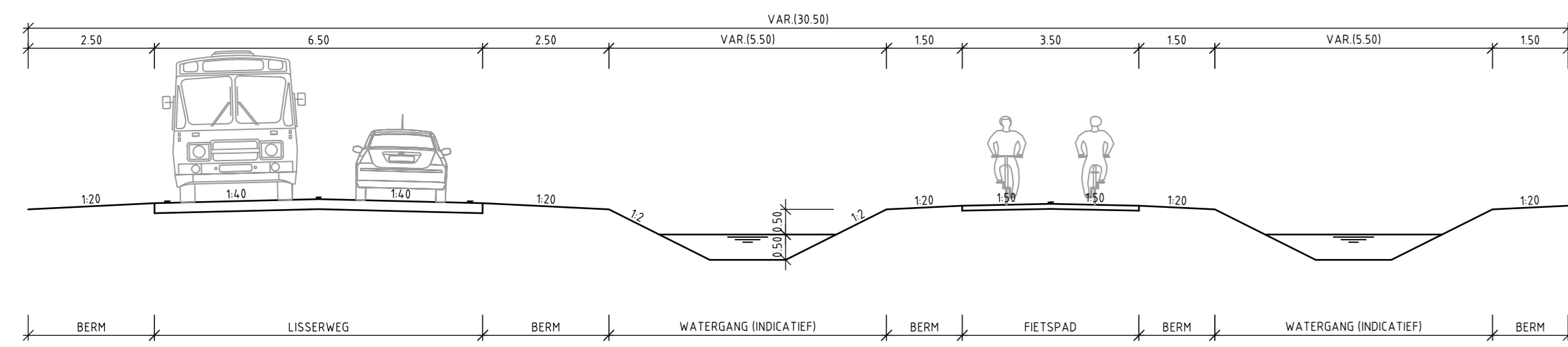
PRINCIPEPROFIEL 1A PROFIEL T.H.V. LIJSSEWEG SCHAAL 1:100
