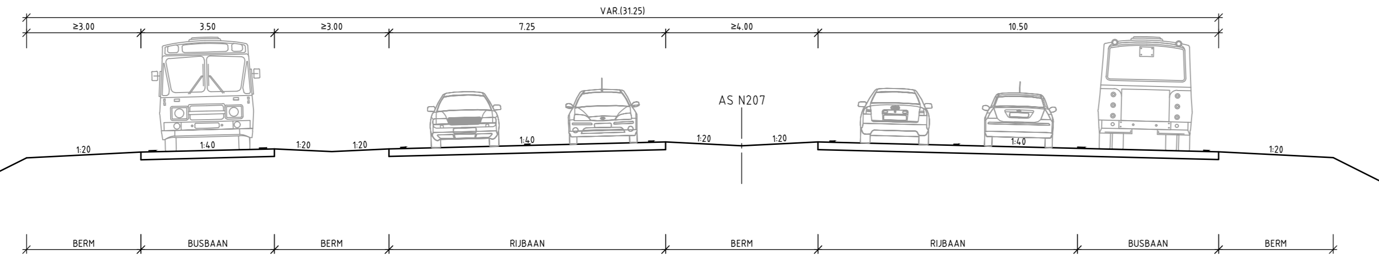
PRINCIPEPROFIEL 2A SCHAAL 1:100 PROFIEL PARALLEL OP OF AAN N207
