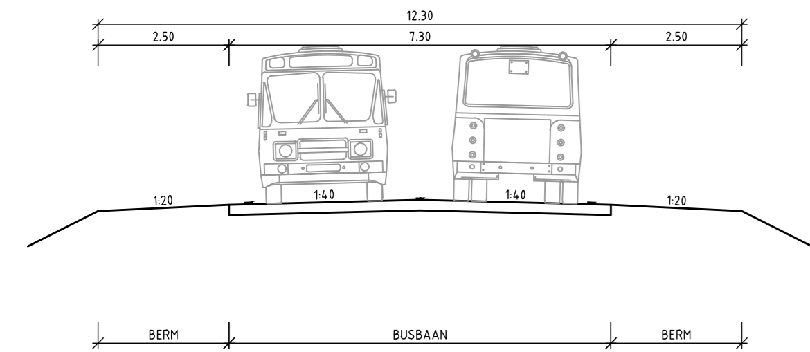
PRINCIPEPROFIEL 1A SCHAAL 1:100 PROFIEL DOOR WOONGEBIED TEN NOORDEN VAN LISSERWEG - IJWEG
