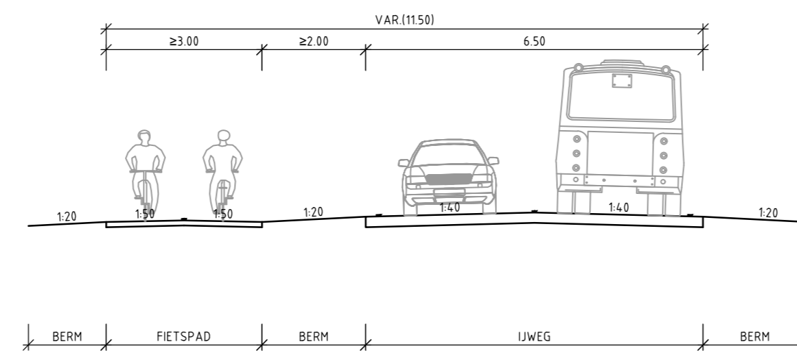
PRINCIPEPROFIEL 2A PROFIEL T.H.V. IJWEG SCHAAL 1:100
