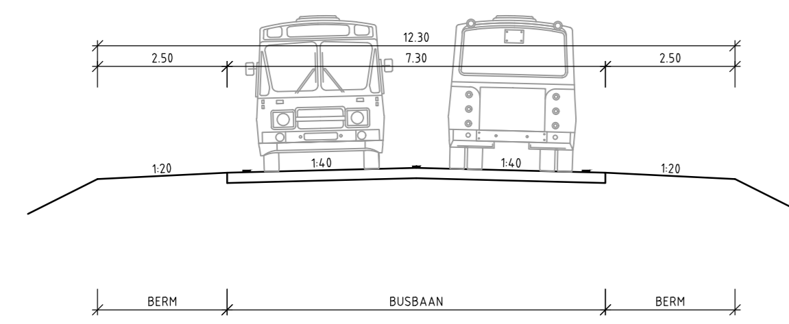
PRINCIPEPROFIEL 1A SCHAAL 1:100 PROFIEL DOOR WOONWEG TEN NOORDEN VAN LISSERWEG - IJWEG
