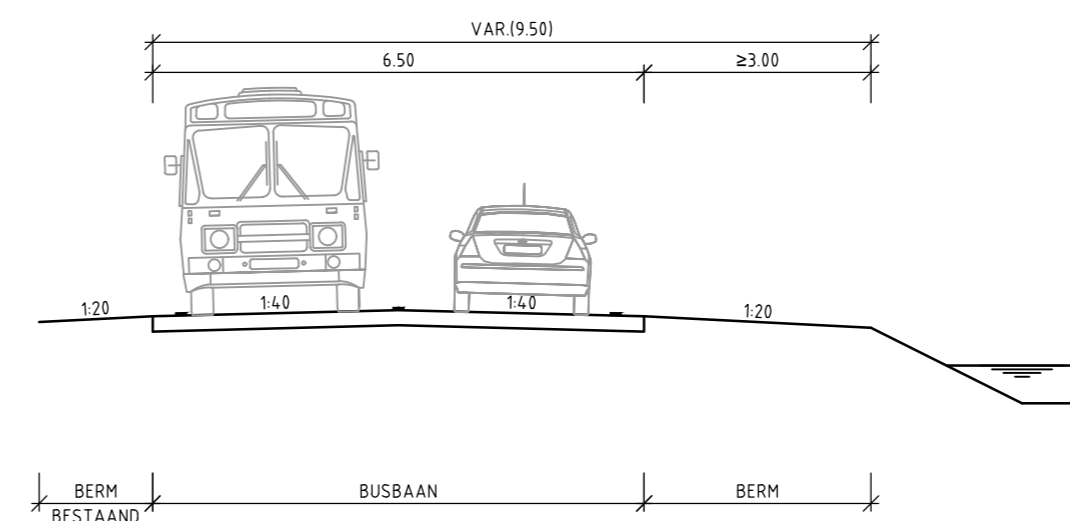
PRINCIPEPROFIEL 3A PROFIEL T.H.V. GETSEWOUDWEG SCHAAL 1:100
