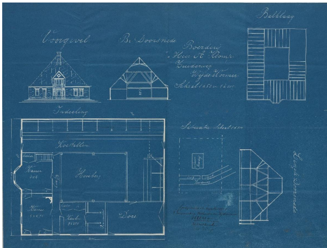
Technische tekening/blauwdruk van een stolpboerderij van de Heer A. Klomp aan de Zuiderweg in Wijde Wormer, 1928. Collectie Provinciale Atlas
