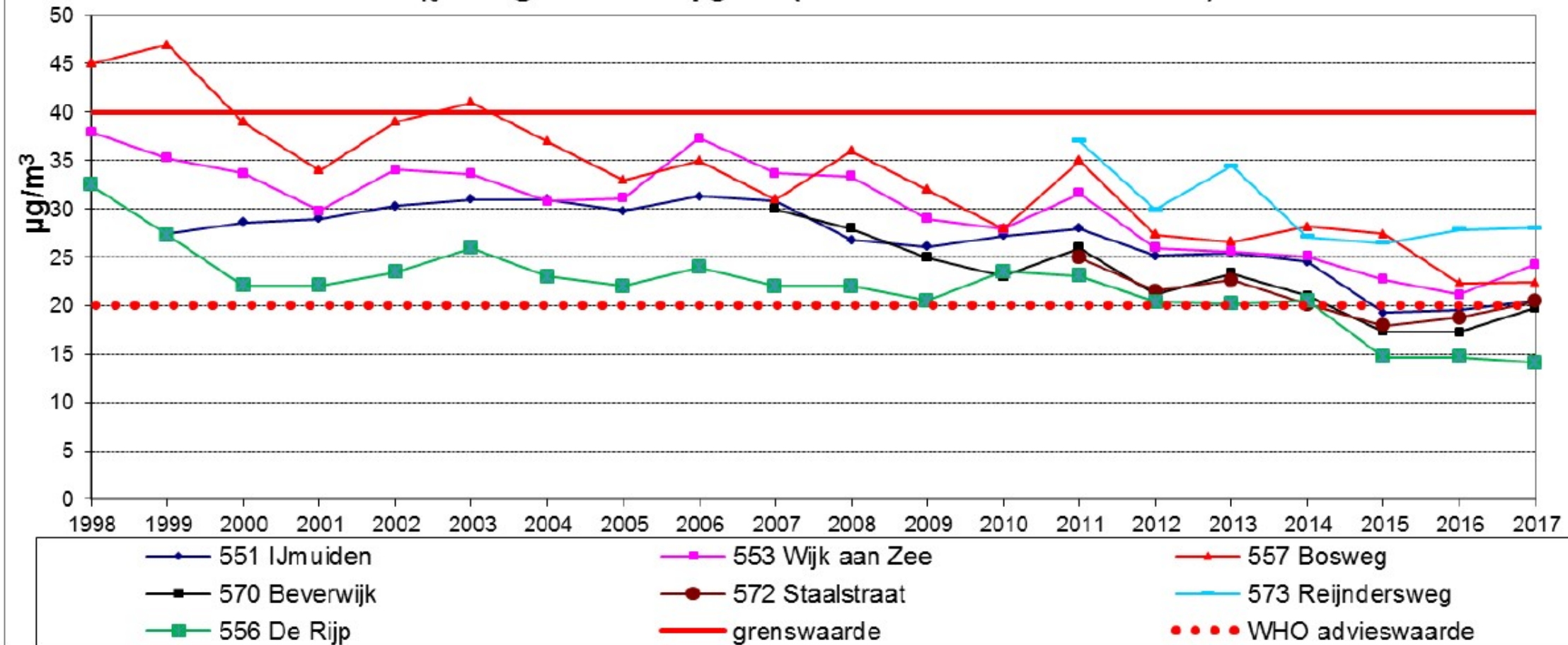
PM 10 Jaargemiddelde \mu\text{g}/\text{m}^3 (exclusief zeezout correcties)
