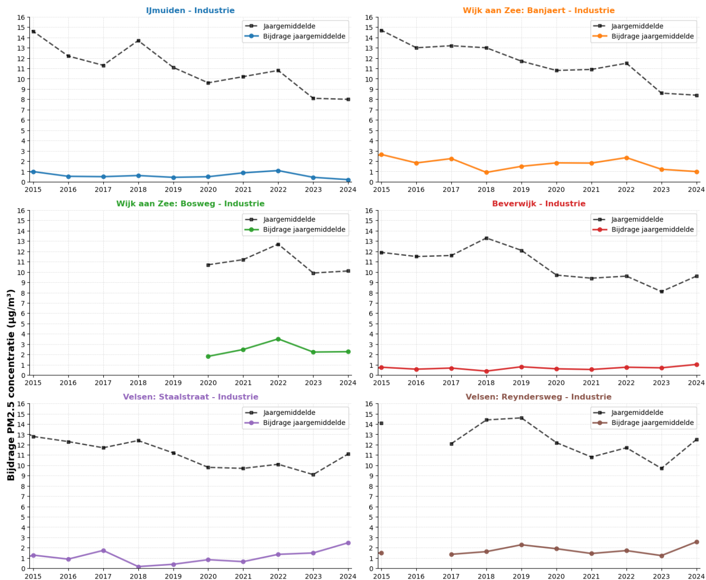
Figuur 18 Concentratiebijdrage bij wind vanaf de industrie in de IJmond (gekleurde lijnen) en totale concentratie op meetstations (zwarte lijnen)
