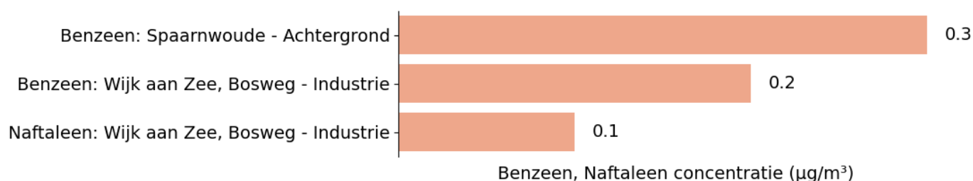
Figuur 24 Jaargemiddelde benzeen en naftaleen concentratie
