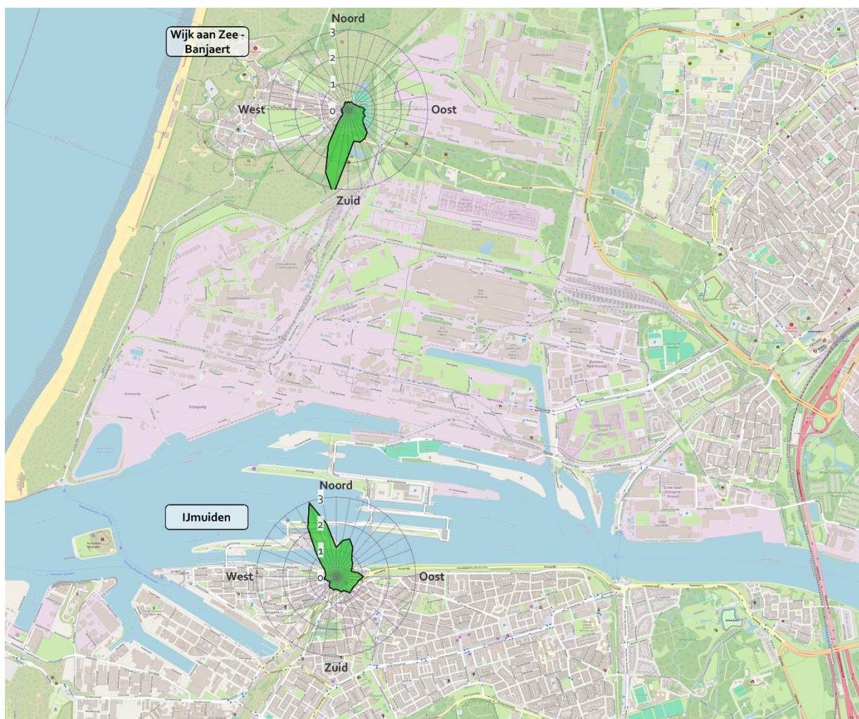
Figuur 32 Jaargemiddelde H_2S concentratie ( \mu g/m^3 ) per windrichting in 2024 op de meetstations (groen).
