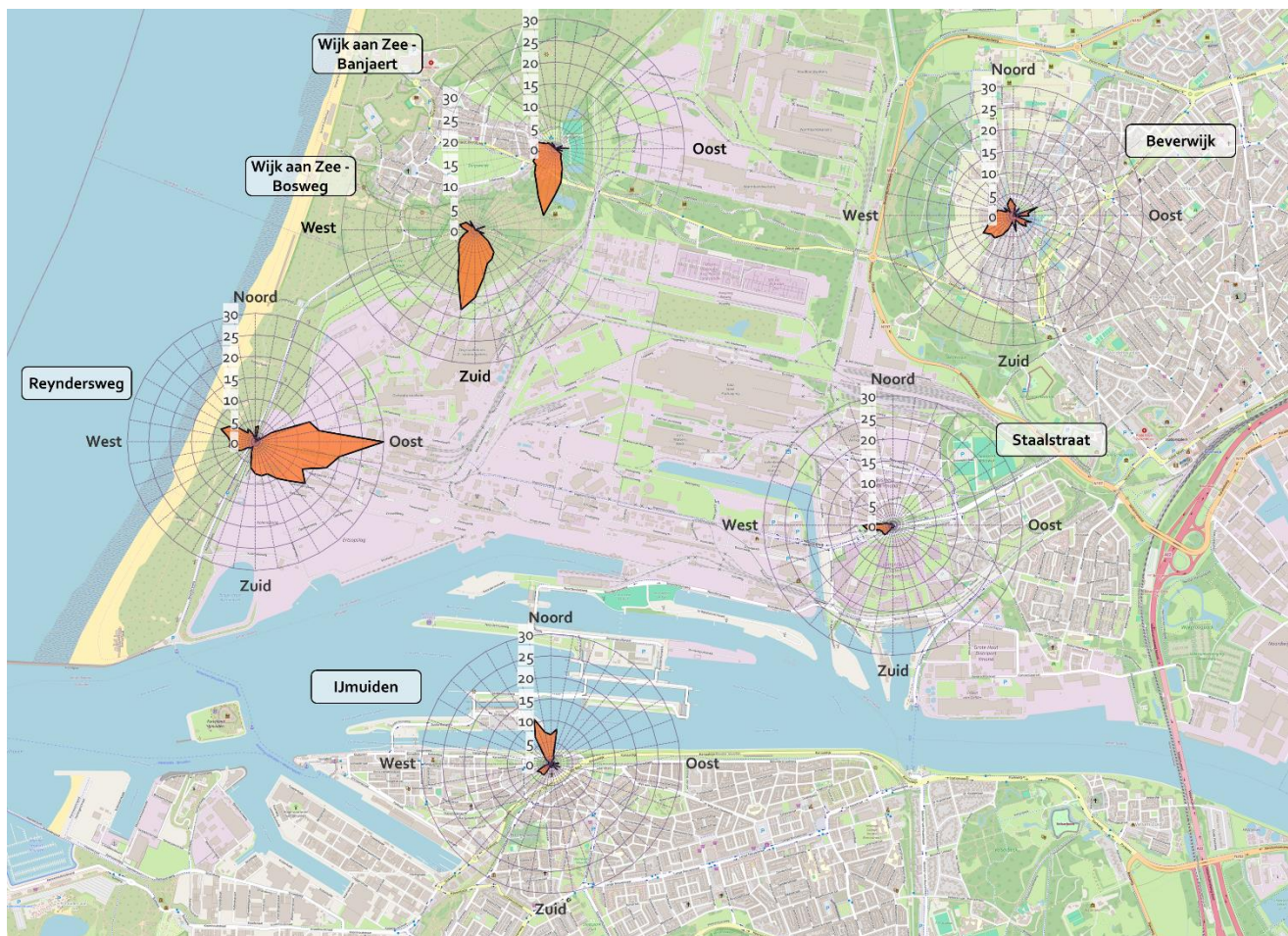
Figuur 12 Versil tussen gemiddelde PM 10 concentratie (µg/m 3 ) op de meetstations en op de achtergrondstations per windrichting in 2024.
