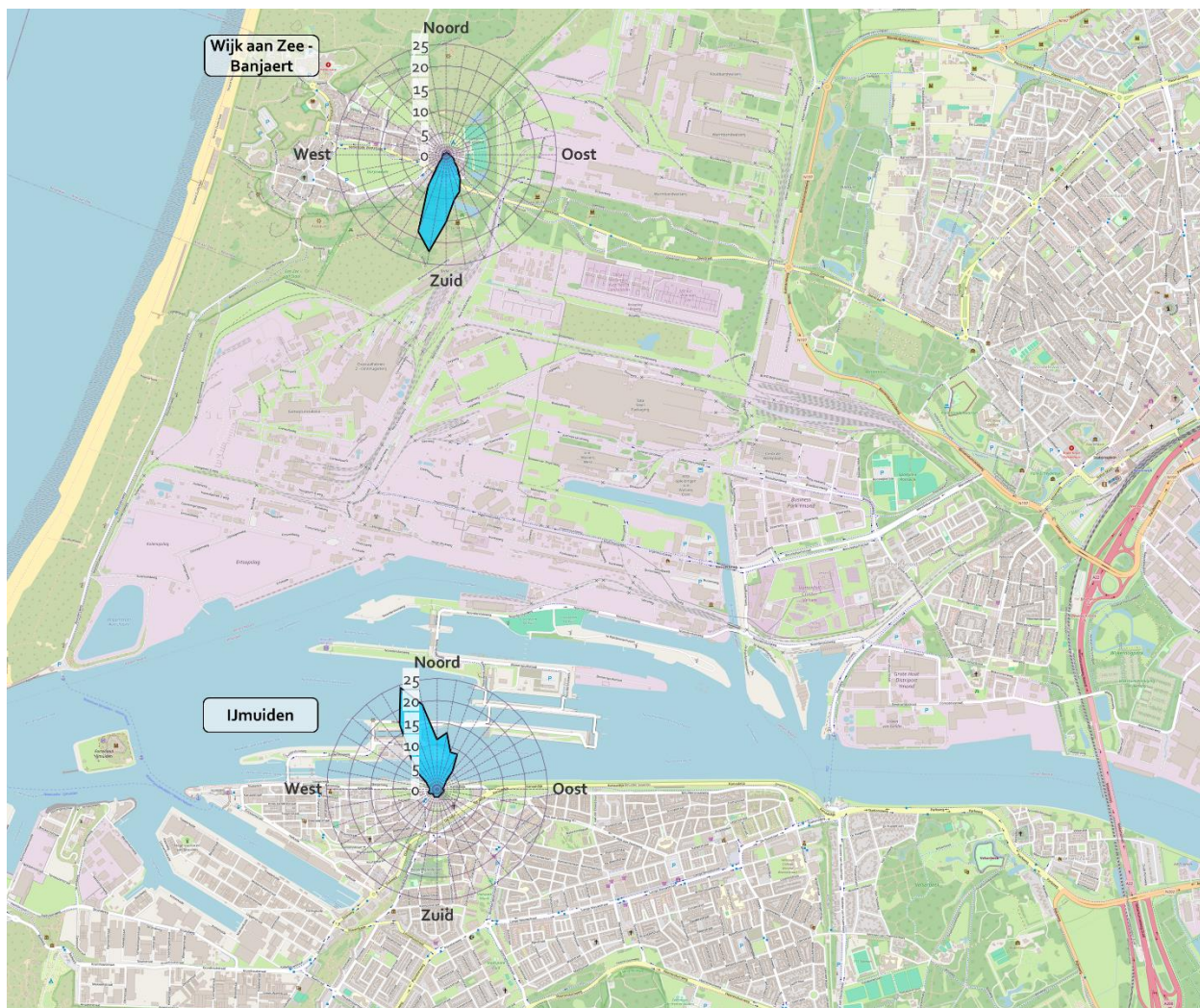
Figuur 29 Jaargemiddelde SO_2 concentratie ( \mu g/m^3 ) per windrichting in 2024 op de meetstations (blauw).
