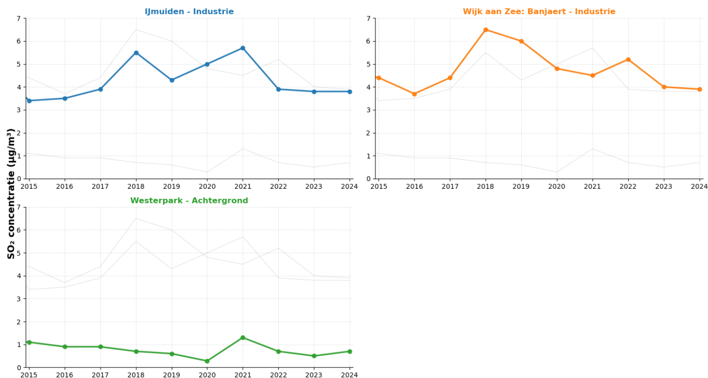
Figuur 28 Trend jaargemiddelde SO 2 concentratie in de afgelopen 10 jaar. De licht grijze lijnen tonen ter vergelijking de resultaten van de andere meetstations.
