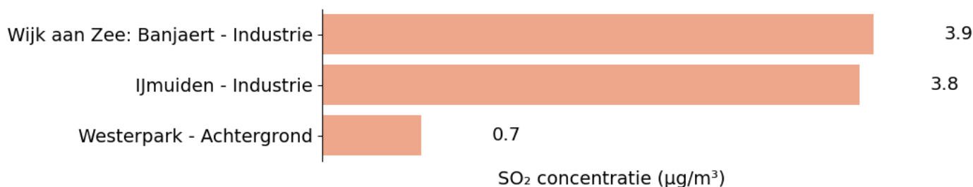
Figuur 27 Jaargemiddelde SO 2 concentratie
