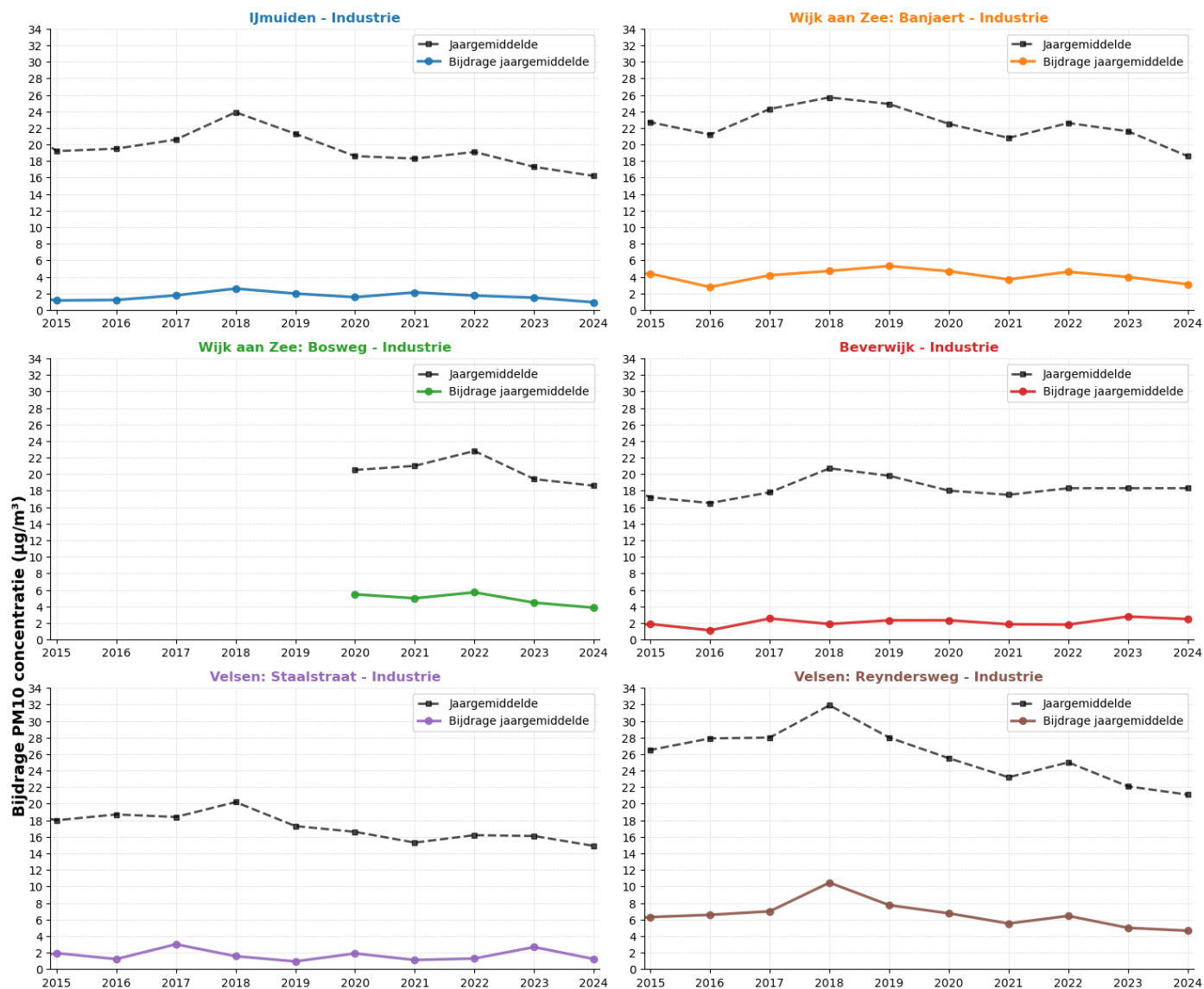
Figuur 13 Concentratiebijdrage bij wind vanaf de industrie in de IJmond (gekleurde lijnen) en totale concentratie op meetstations (zwarte lijnen).
