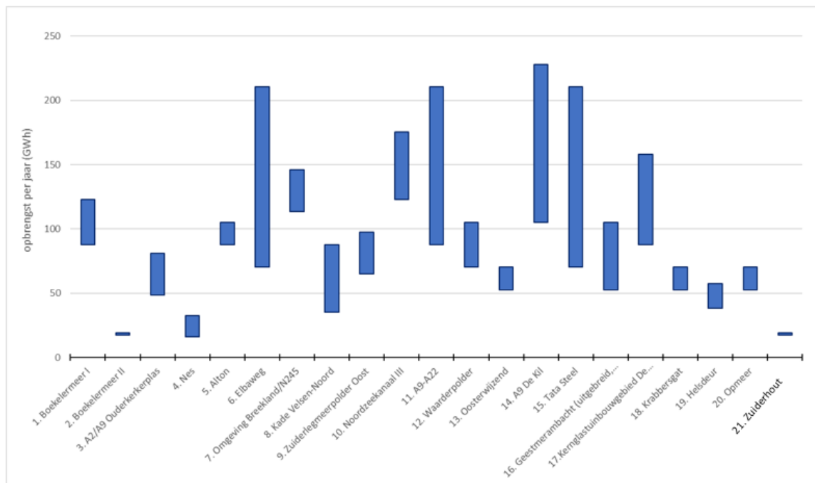
Figuur 9-5 Indicatie van de energieopbrengst voor de zoekgebieden RES 2024. De bandbreedte wordt veroorzaakt door de inschatting van het minimum en maximum aantal turbines per zoekgebied
