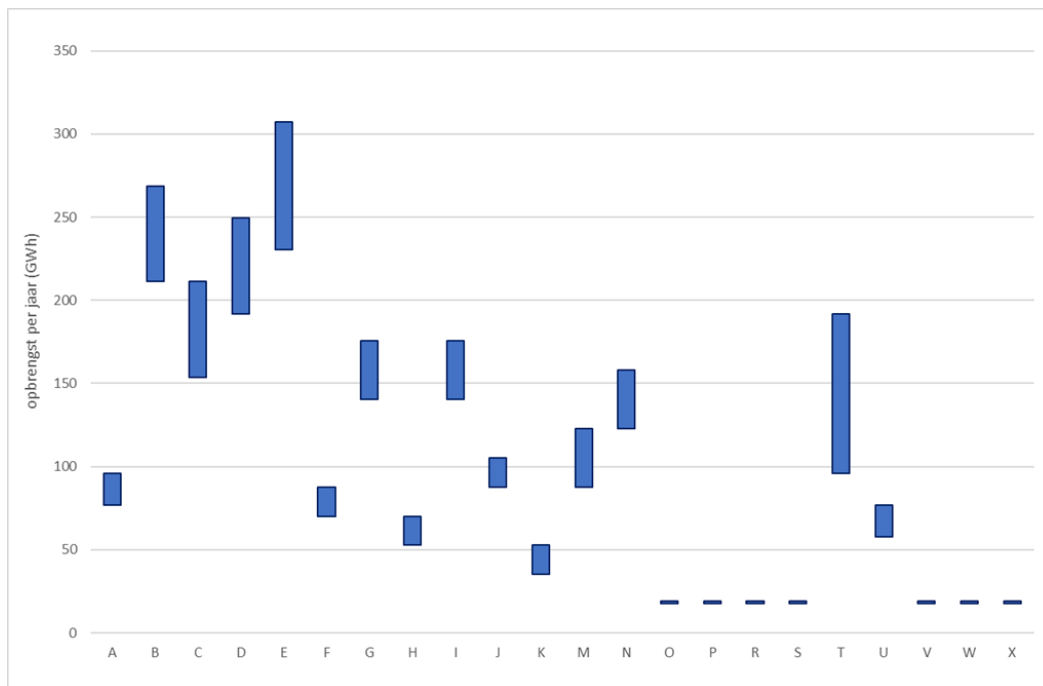
Figuur 11-27 Indicatie van de energieopbrengst voor de potentiële gebieden op termijn. De bandbreedte wordt veroorzaakt door de inschatting van het minimum en maximum aantal turbines per locatie
