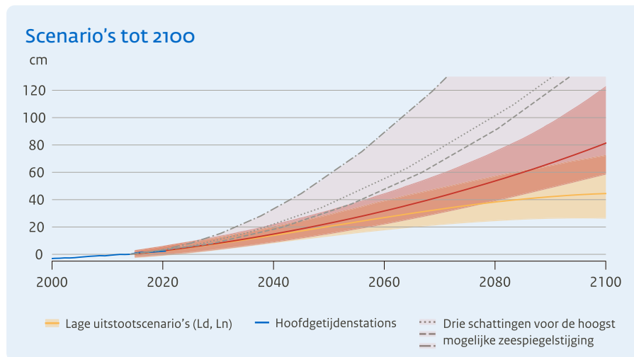
Figuur 3: Scenario's zeespiegelstijging voor de Nederlandse kust tot 2100, uit KNMI'23 klimaatscenario's
