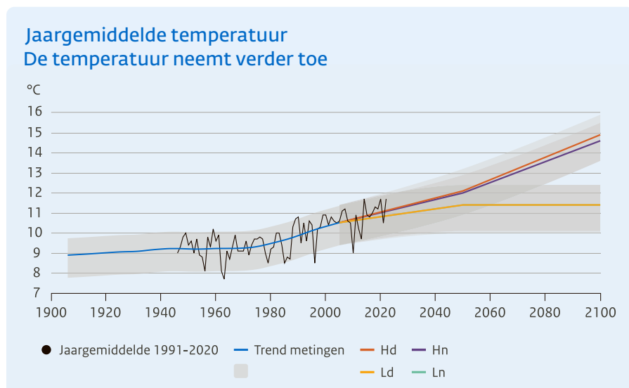
Figuur 4: Jaargemiddelde temperatuur in Nederland in 2050 en 2100, uit KNMI'23 klimaatscenario's
