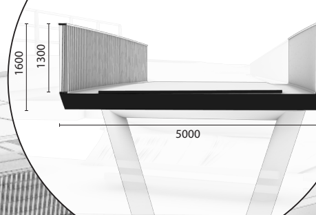
Principeddoorsnede brugdek met maatvoering
