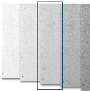
Schoonbeton conform CUR100 klasse B1 civiel
