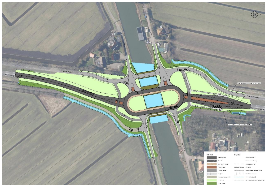
Afbeelding 1: schets ovonde Beets
