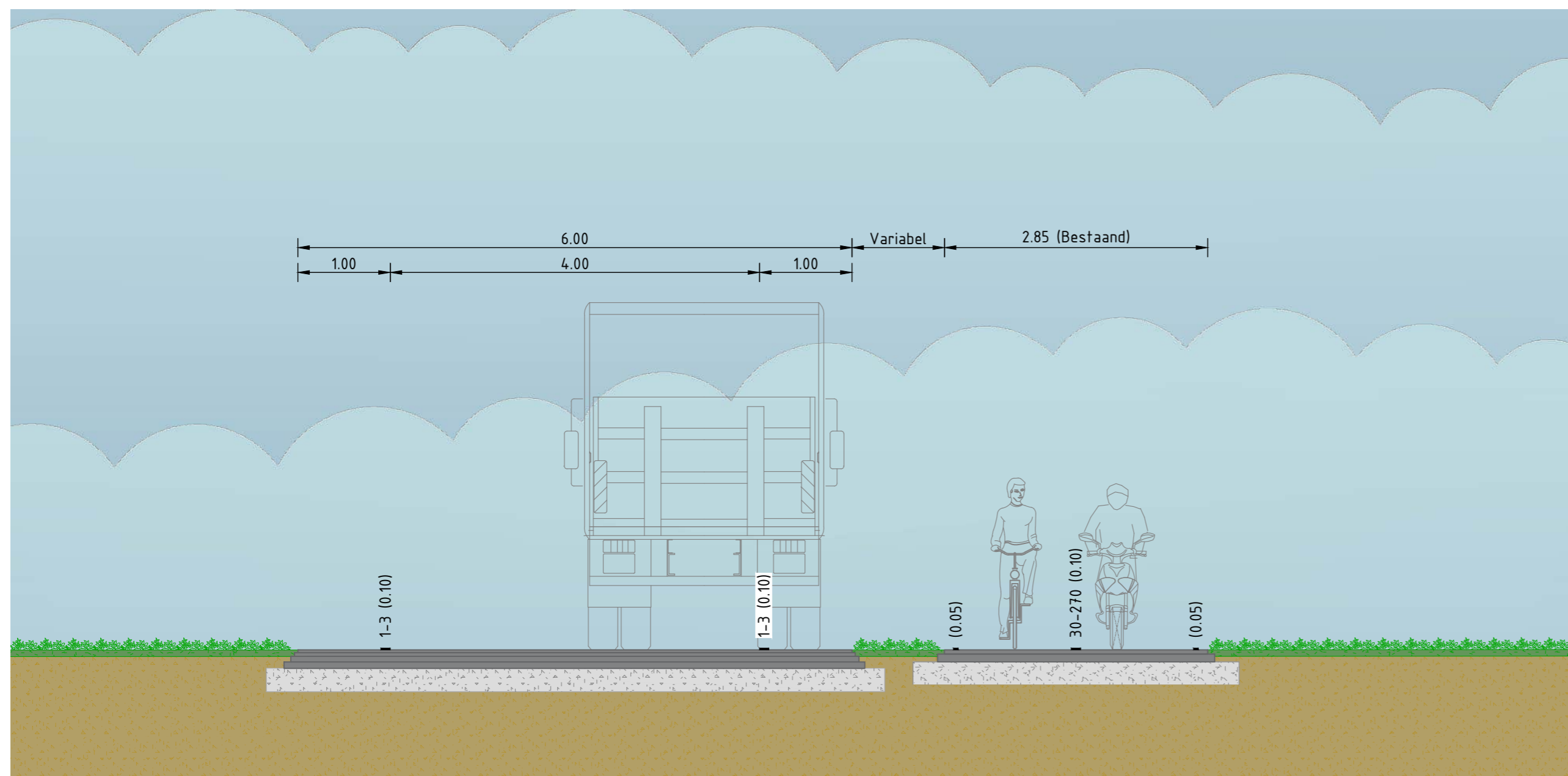
PRINCIPEPROFIEL B ETW60 (Buiten de bebouwde kom) SCHAAL 1 : 50
