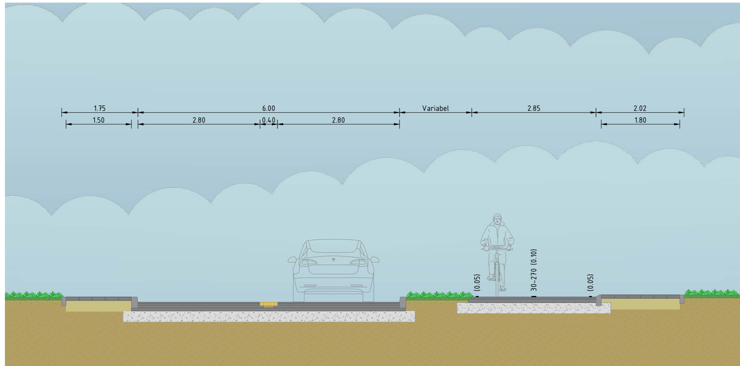
PRINCIPEPROFIEL A GOW50 (Binnen de bebouwde kom) SCHAAL 1 : 50
