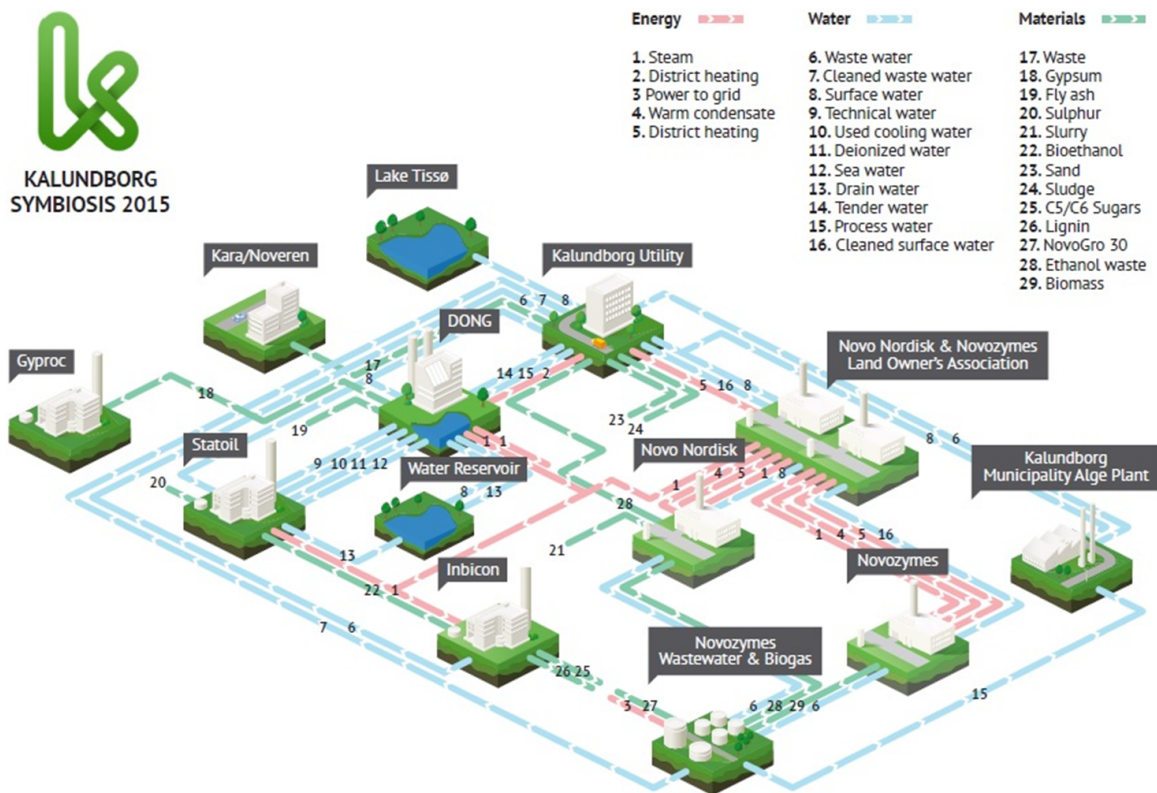
Figuur: Schema van de bestaande industriële symbiose op het bedrijventerrein van Kalundborg in Denemarken
